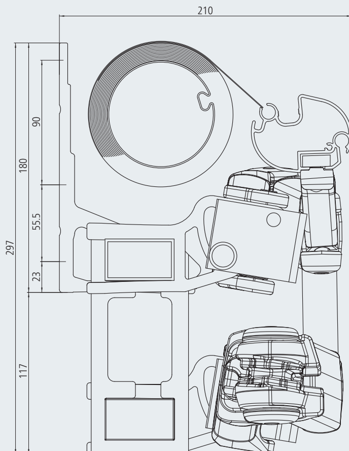
Querschnitt Topas MiniMax ohne Dach
