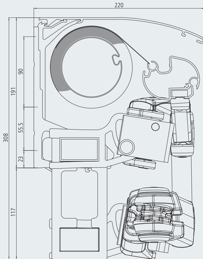
Querschnitt Topas MiniMax mit Dach
